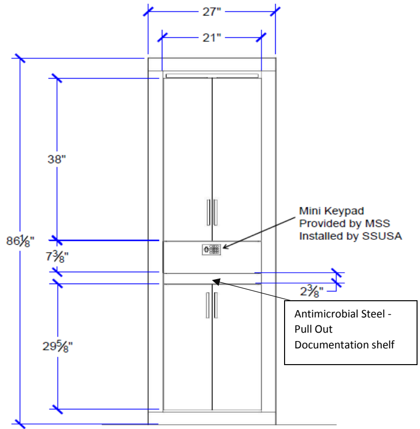
1 FRONT SS-1 SCALE: 1/2" = 1'0"
